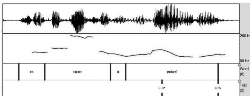
Figura 9. Forma d'onda, curva di f_0 e trascrizione ToBI del contorno nucleare della DS Sei capace di guidare? prodotta dall'informatore GT.
