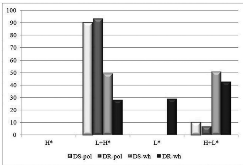
Figura 6. Percentuali di ricorrenza (%) degli accenti intonativi.
