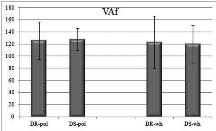
Figura 3. Durata media e deviazione standard (ms) di VAF.
