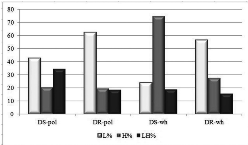
Figura 5. Percentuali di ricorrenza (%) dei toni di confine.
