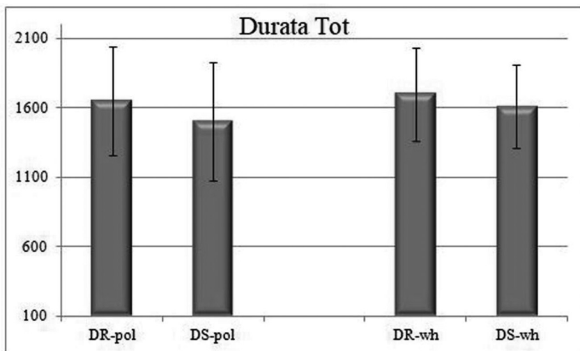
Figura 1. Durata totale media e deviazione standard (ms).
