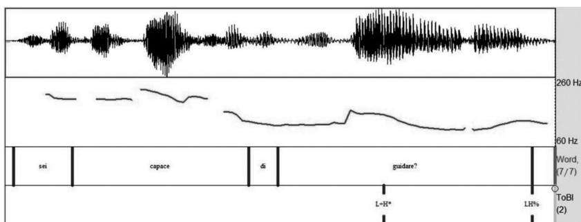
Figura 10. Forma d'onda, curva di f_0 e trascrizione ToBI del contorno nucleare della DR Sei capace di guidare? prodotta dall'informatore GT.
