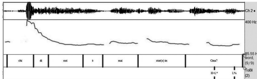
Figura 8. Forma d'onda, curva di f0 e trascrizione ToBI del contorno nucleare della DR Chi di noi è mai stato in Cina? prodotta dall'informatrice G3.
