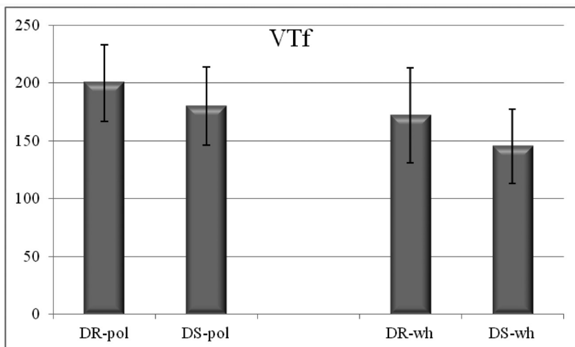
Figura 2. Durata media e deviazione standard (ms) di VTf.
