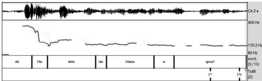
Figura 11. Forma d'onda, curva di f_0 e trascrizione ToBI del contorno nucleare della DR Chi l'ha detto che Marisa si sposa? prodotta dall'informatrice FC.
