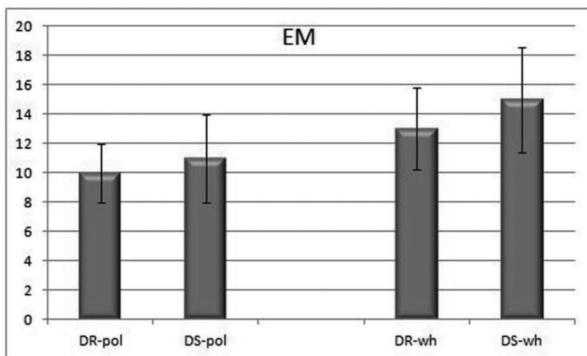
Figura 4. Escursione melodica media e deviazione standard (ST).
