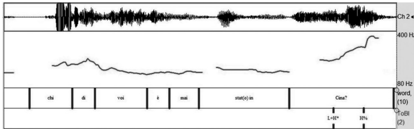
Figura 7. Forma d'onda, curva di f0 e trascrizione ToBI del contorno nucleare della DS Chi di voi è mai stato in Cina? prodotta dall'informatrice G3.
